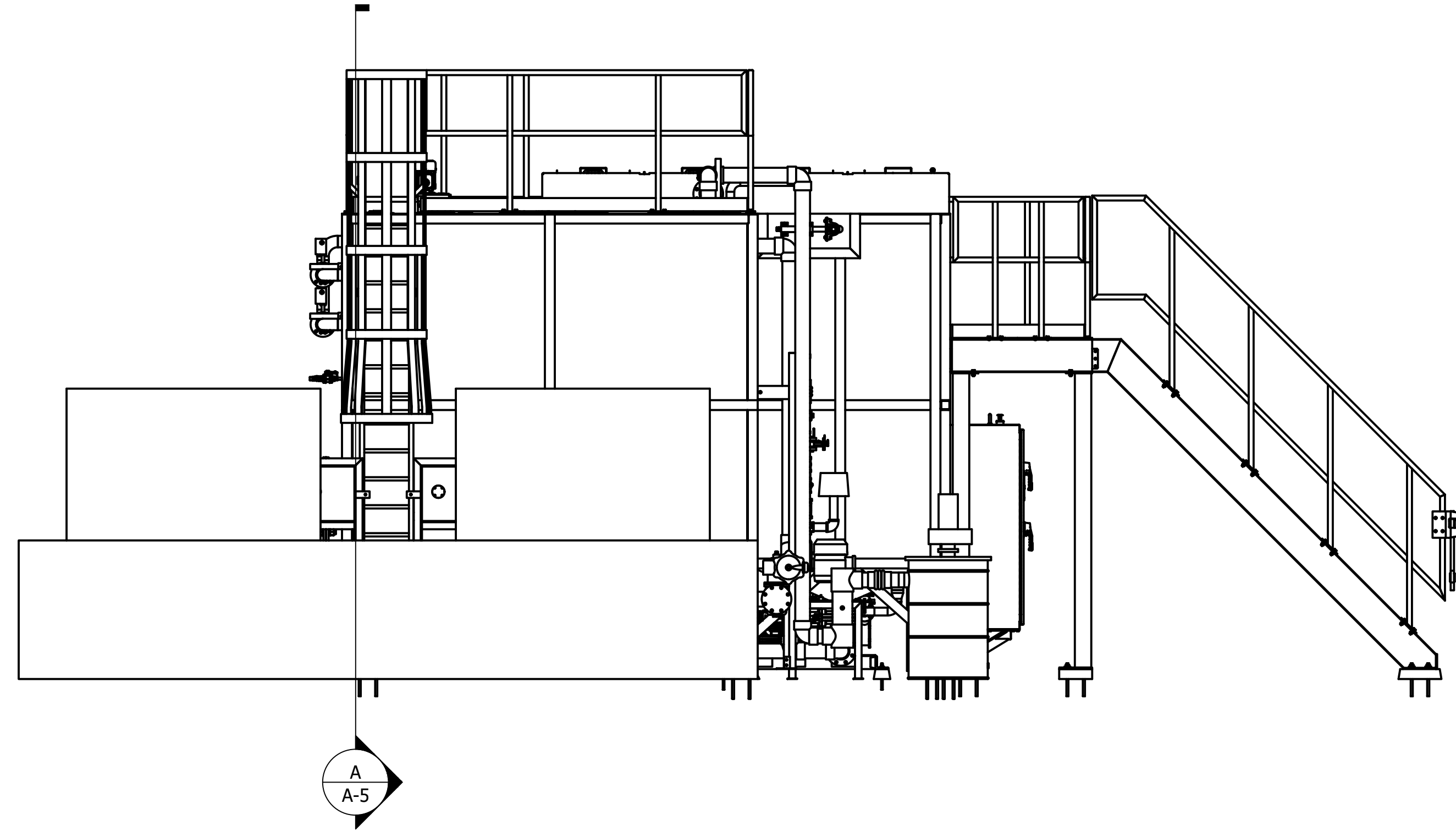
3 LEFT VIEW Scale: 3/8" = 1'-0"
